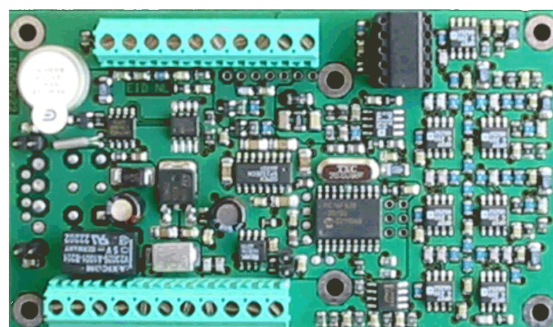
LID 650 OEM-Board
